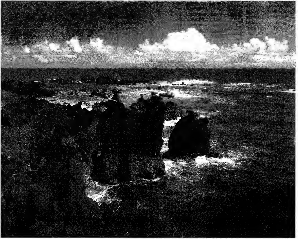
صورة لتآكل شواطئ البحار بفعل الأمواج
